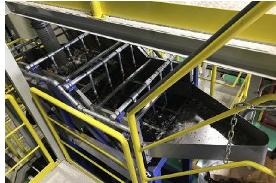
湿式比重差選別機
