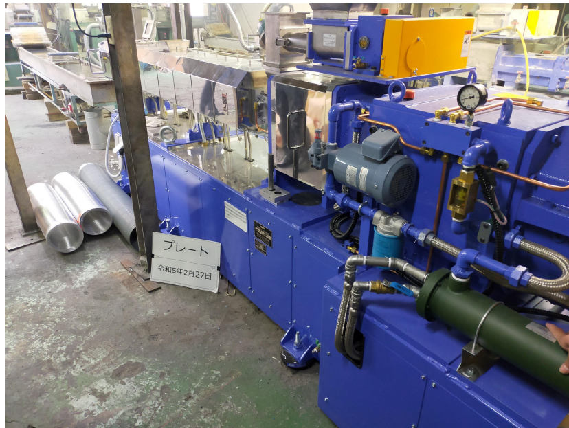
二軸押出機
