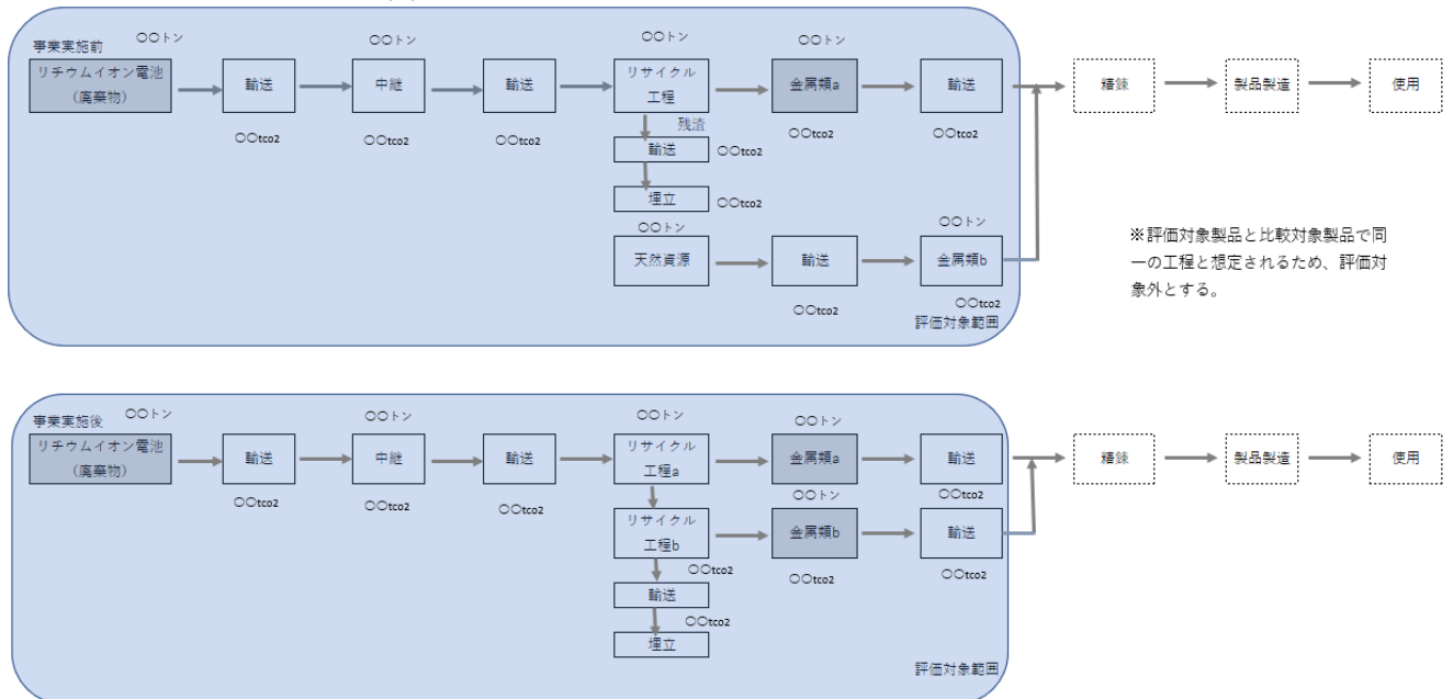
リチウムイオン電池リサイクルフロー図（例）
