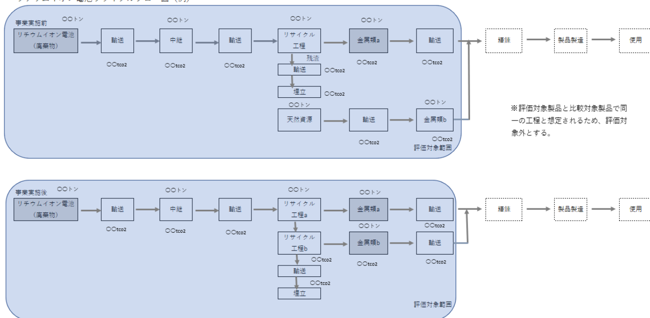
リチウムイオン電池リサイクルフロー図（例）
